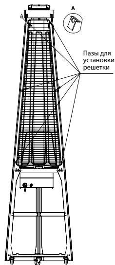
Рис. 4 – Установка решетки
