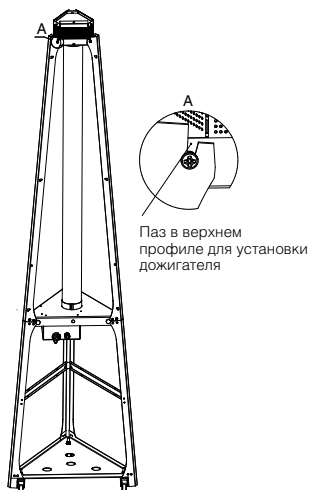
Рис. 3 – Установка колбы и дожигателя
