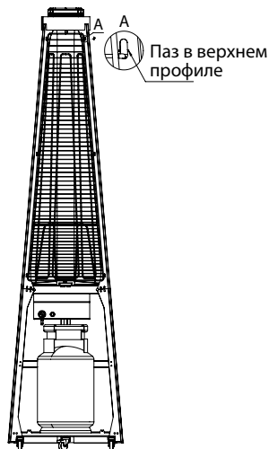
Рис. 5 – Установка фиксаторов решетки
