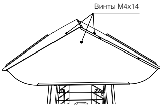
Рис. 7 – Установка козырька
