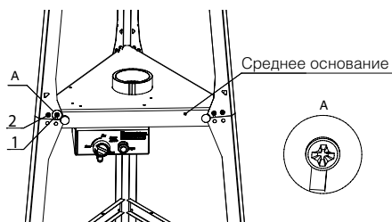
Рис. 1 – Установка верхних профилей
